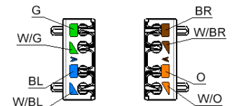
Anschlussbelegung / PIN assignment T568A nach / according to TIA-568.2-D
