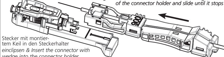
Siehe Steckerhalter Bild 4 See connector holder picture 4
