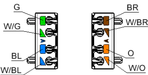
Anschlussbelegung / PIN assignment T568B nach / according to TIA-568.2-D
